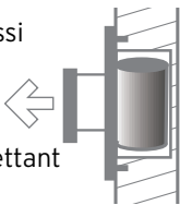
Beltrac Mural M / L (Encastrable) sangle 2,3 m / 3,7 m
